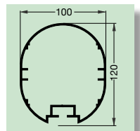
Jugendfussballtor 5 x 2 m zerlegbar aus ovalem Aluminium-Profil 100 x 120 mm, eloxiert, Gehrungen verschweisst, Bodenrahmen 80 x 40 mm, nach Vorschrift des SFV. 02100 Stück 1'380.-
