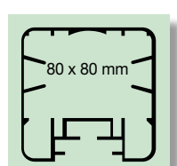
Jugendfussballtor 5 x 2 m „Schule“ freistehend, aus Aluminium-Profil 80 x 80 mm. Netzbügel und Bodenrohr aus verzinktem Stahlrohr. 56108 Torrahmen silber Stück 1'150.-
