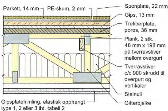
Fig. 3 Etasjeskiller med golvtype 2
