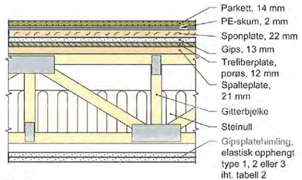
Fig. 4 Etasjeskiller med golvtype 3
