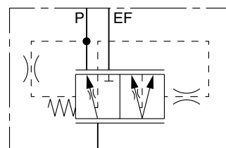
Prioritätsventil Funktion „A“ max. Volumenstrom
