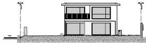
SÜDFASSADE 1:100
